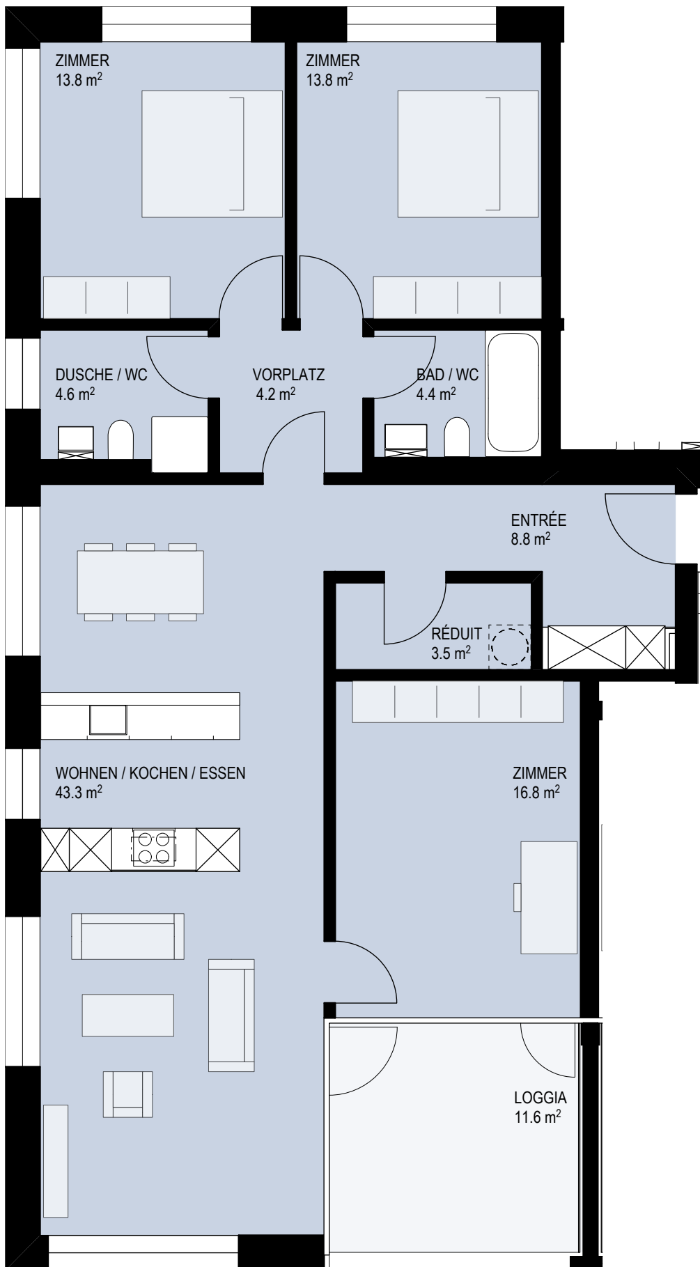
E.601: 4.5-Zimmer-Wohnung NWF: 113.2 m 2 / Loggia 11.6 m 2
